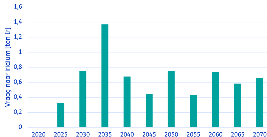
Jaarlijkse vraag naar virgine iridium voor PEM elektrolyserproductie in de EU
